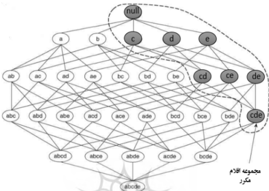
شکل ۴. تصویری از اصول الگوریتم Apriori (Tan 2006)
