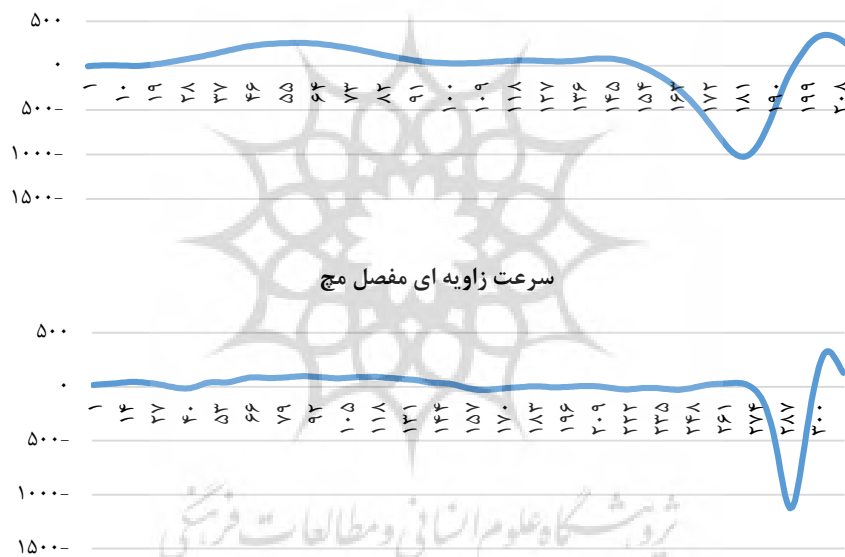
شکل ۱- نمودار سرعت زاویه‌ای مفصل آرنج و میچ مرتبط با مراحل مختلف الگوی اجرا
