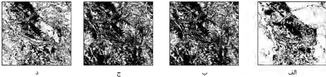
شکل ۵. نقشه تغییرات به دست آمده از تکنیک‌های موجک، تفاضل، نسبت و طبقه‌بندی (رنگ مشکی: مناطق دارای تغییر، رنگ سفید: مناطق بدون تغییر). الف) تکنیک موجک، ب) تفاضل، ج) نسبت، د) طبقه‌بندی
