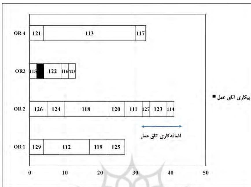
شکل ۳. نمودار گانت نتایج الگوریتم ژنی و همکاران در حل یک مسئله نمونه
