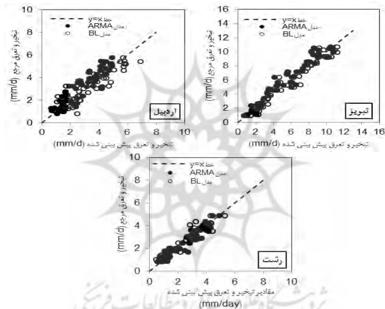
شکل (۲) مقایسه مقادیر پیش‌بینی شده ET+ توسط مدل‌های خطی و غیرخطی با مبنای قرار دادن مقادیر تبخیر و تعرق مرجع در مرحله صحت‌سنجی (خط چین: خط y=x )
