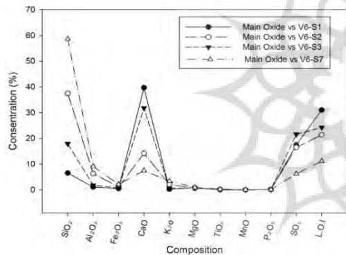
شکل ۱۱: نمودار مقایسه اکسیدهای اصلی نمونه‌های مورد مطالعه با استفاده از تجزیه شیمیایی XRF (W%)
