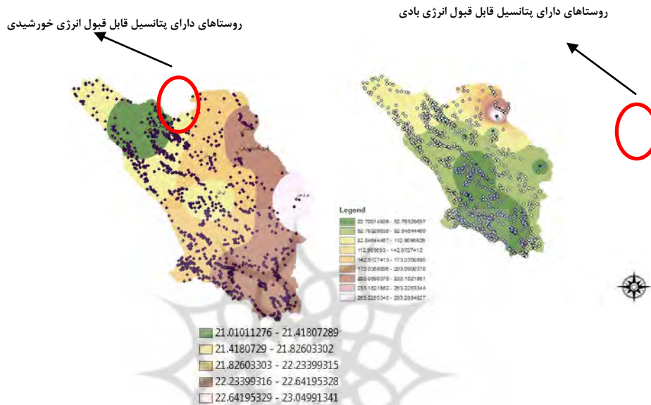
شکل شماره (۲) نقشه پراکندگی روستاهای استان چ و ب با محوریت پهنه انرژی خورشیدی: مگاژول بر متر مربع (منبع: یافته‌های تحقیق)
