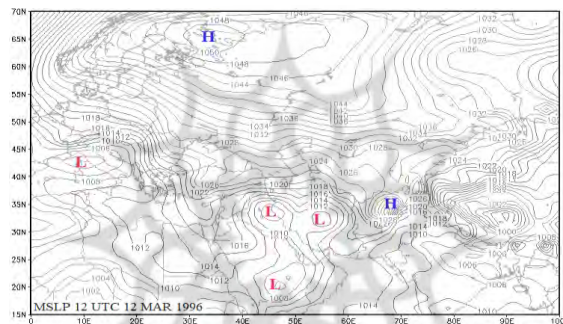
شکل ۱۰- نقشه هم‌دیدی فشار در سطح متوسط دریا مربوط به ساعت ۱۲ UTC روز ۱۲ ام مارس ۱۹۹۶.
