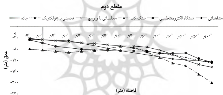
شکل ۶. مقایسه مطالعات مختلف تعیین حد تداخل آب شور و شیرین در مقطع دوم نوره
