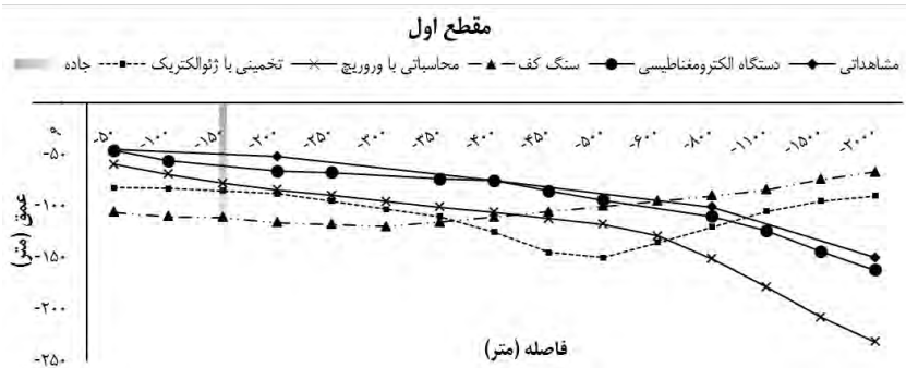
شکل ۵. مقایسه نتایج مطالعات مختلف تعیین حد تداخل آب شور و شیرین در مقطع اول نوره
