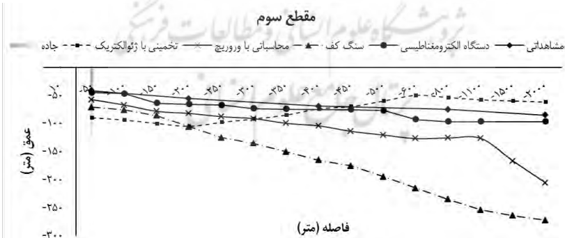
شکل ۷. مقایسه نتایج مطالعات مختلف تعیین حد تداخل آب شور و شیرین در مقطع سوم نوره
