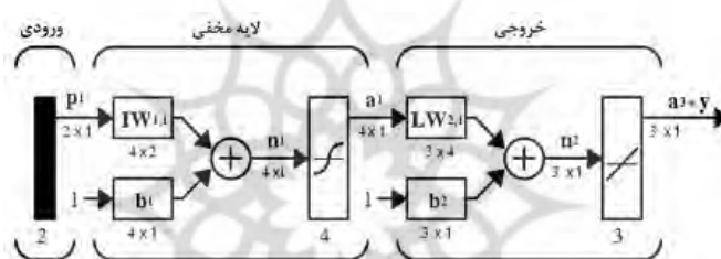
شکل ۶- ساختار پرسپترون چندلایه با نورون‌های پنهان و نورون‌های خروجی با تابع خطی (۳۰)
