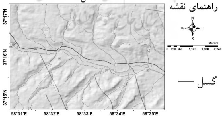
شکل ۸- نقشه گسل های منطقه مورد مطالعه (مأخذ سازمان زمین شناسی کشور)
