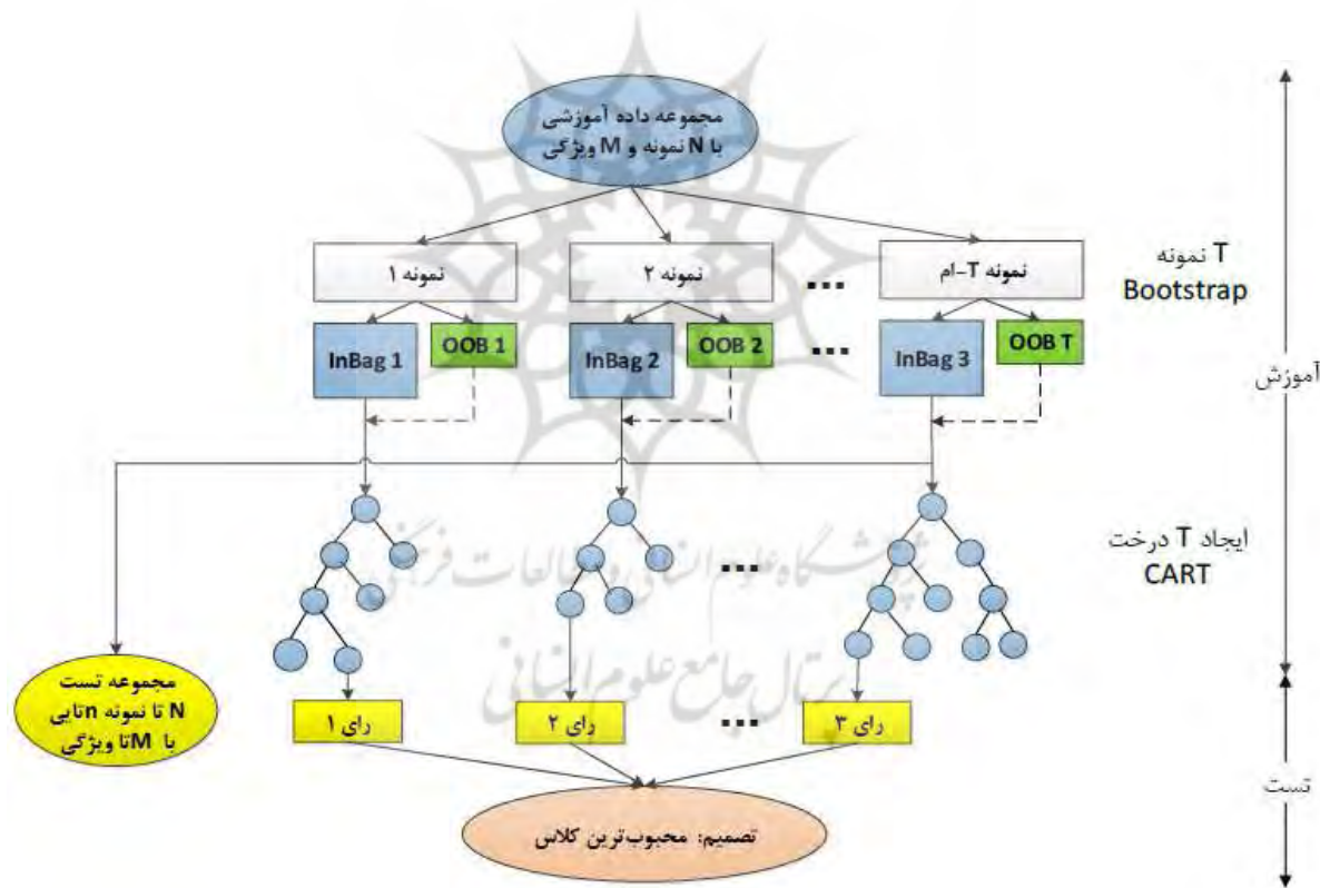
شکل ۵: روند کلی الگوریتم جنگل تصادفی (ژئو و همکاران، ۲۰۱۱)
