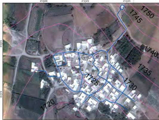
شکل شماره (۸): ترسیم شبکه آب روستا
