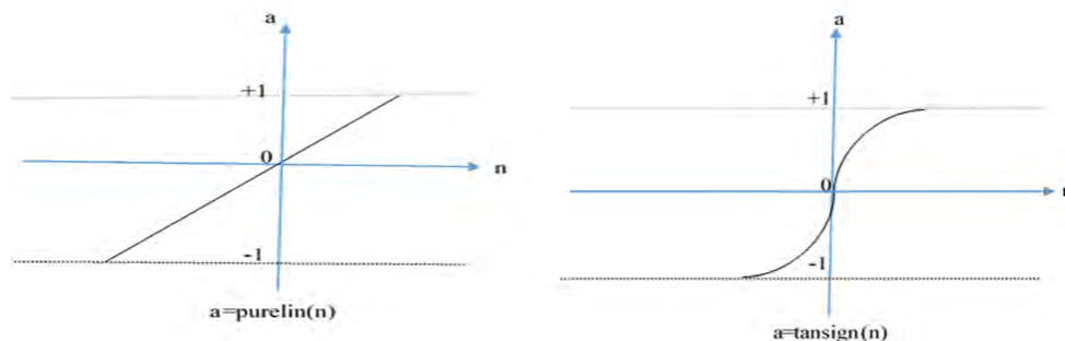
شکل (۶). انواع تابع محرک شبکه‌های پس انتشار
