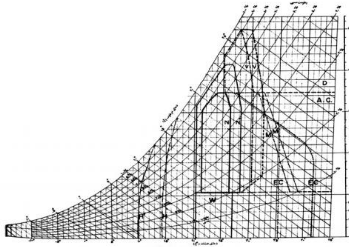
نمودار ۱- زیست اقلیم ساختمانی گیونی (گرچی مهبلیانی و دیگران، ۱۳۹۰، ص.ص. ۴۱-۳۱)
