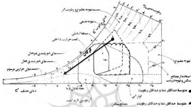
نمودار ۳- سایکرومتریک شهر گرگان اصلاح شده (نگارندگان)
