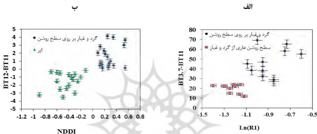
شکل ۳. استخراج حد آستانه‌ها در شاخص‌های مورد استفاده
