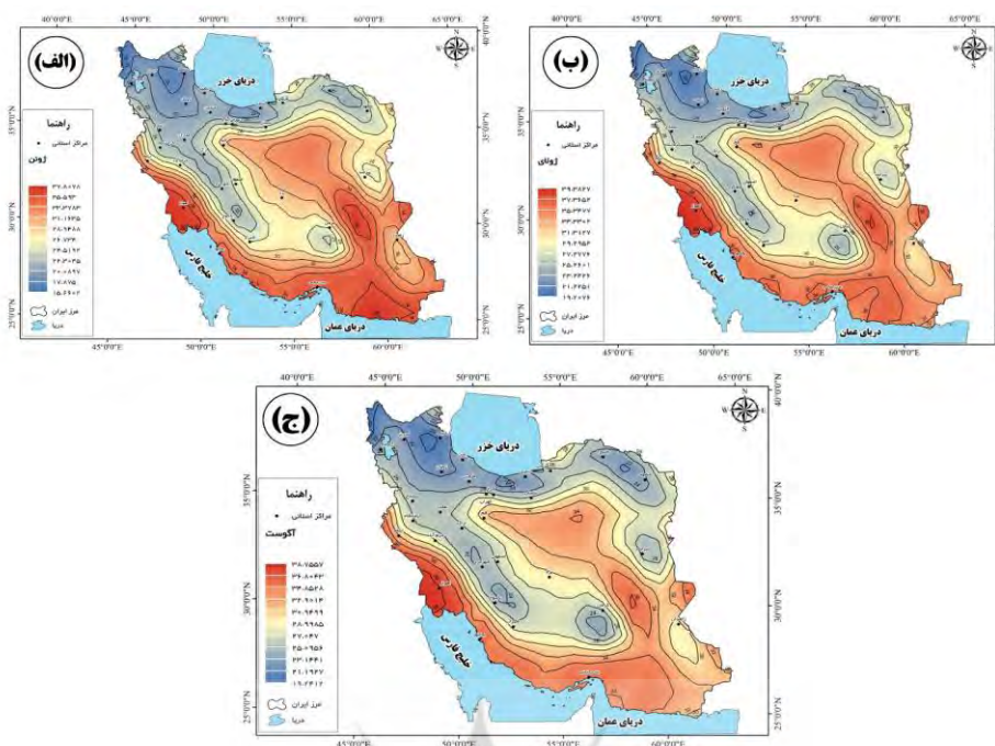
شکل ۵. دمای ماهیانه ایران مبتنی بر برون داد پایگاه پیش‌بینی میان مدت هواسپهر اروپایی (ECMWF) نسخه ERA-Interim؛ (الف) ماه ژوئن؛ (ب) ماه ژوئای؛ (ج) ماه آگوست
