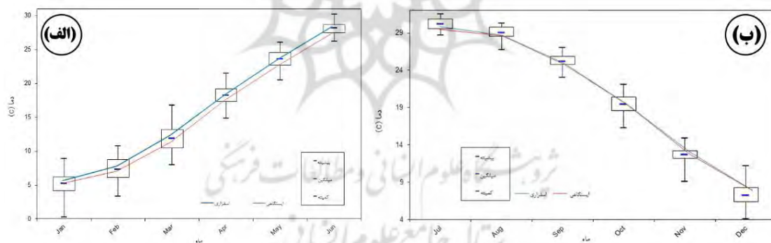
شکل ۲. همسنگی دمای ماهیانه ایران مبتنی بر برون داد پایگاه پیش بینی میان مدت هوا سپهر اروپایی (ECMWF) نسخه - ERA-Interim و دمای پیمونگاهی و پایگاه ملی اسفزاری؛ الف) شش ماهه اول سال؛ ب) شش ماهه دوم سال
