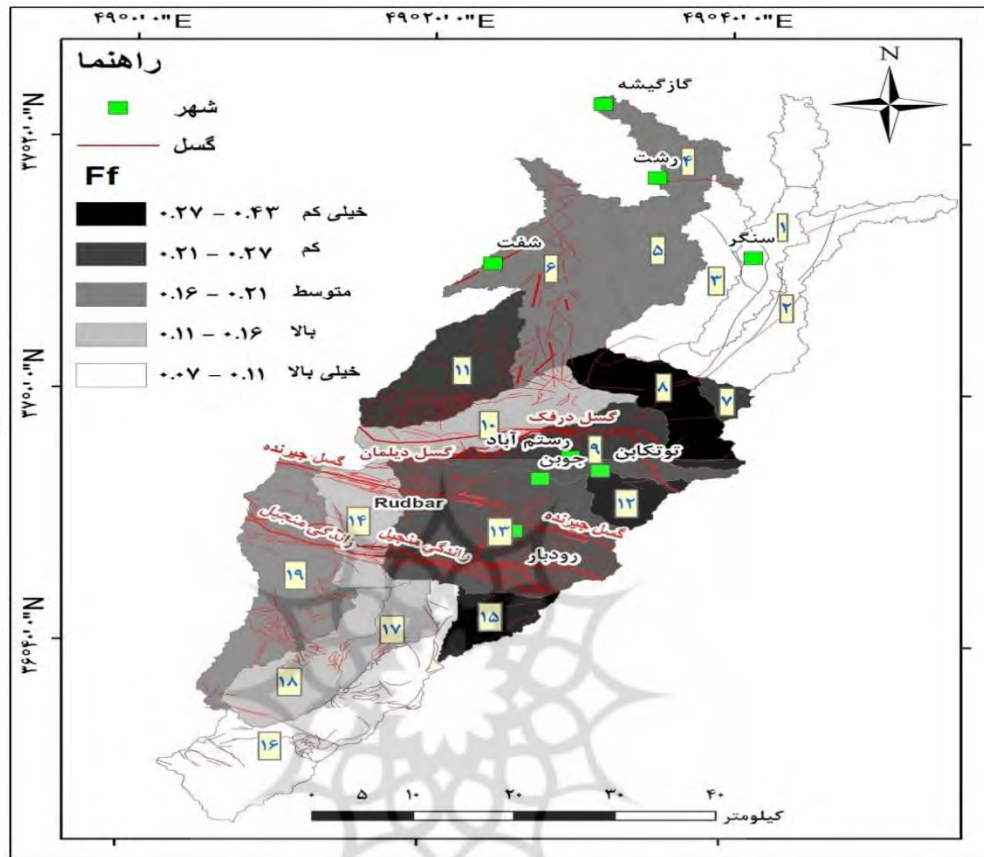
شکل ۱۱: نقشه پراکنندگی شاخص ضریب شکل
