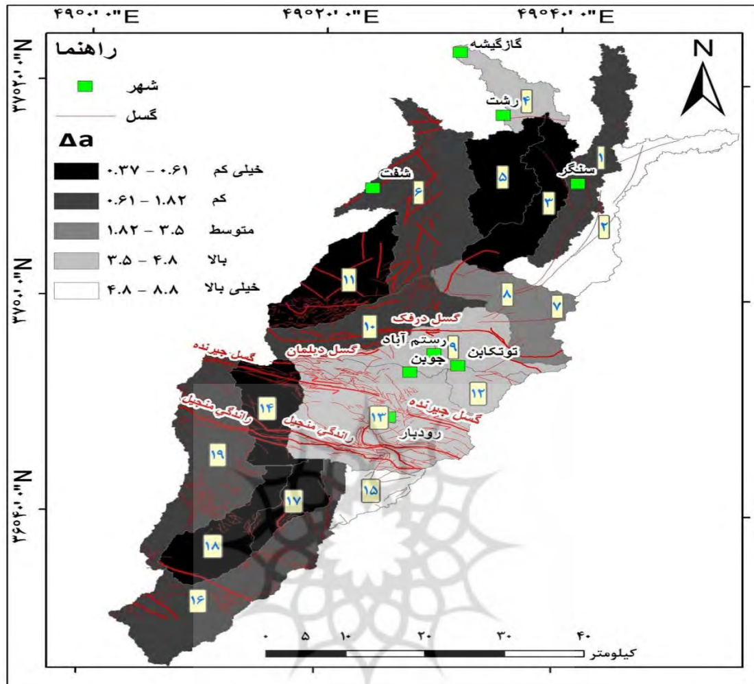
شکل ۵: نقشه‌ی پراکنندگی مقادیر شاخص ناهنجاری سلسله مراتبی در منطقه‌ی مورد مطالعه.
