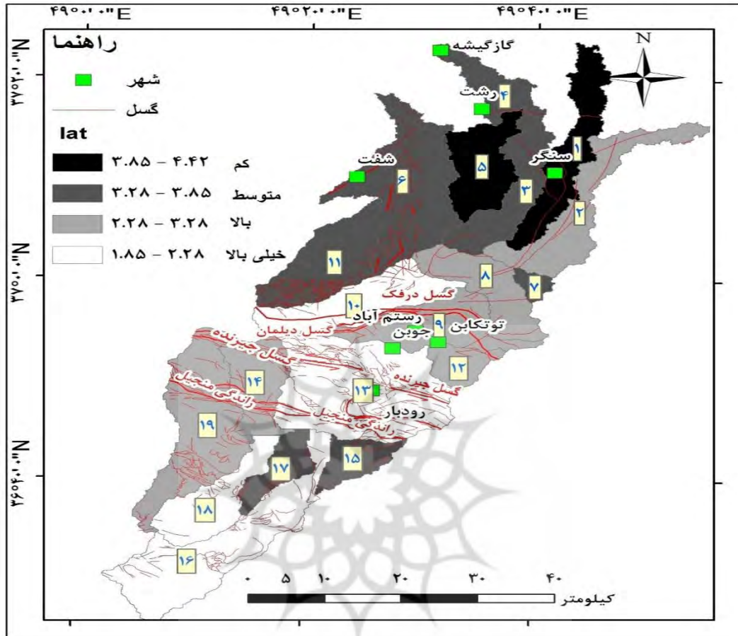
شکل ۱۳: نقشه‌ی توزیع سطح فعالیت زمین‌ساختی نسبی (Iat) در منطقه مورد مطالعه
