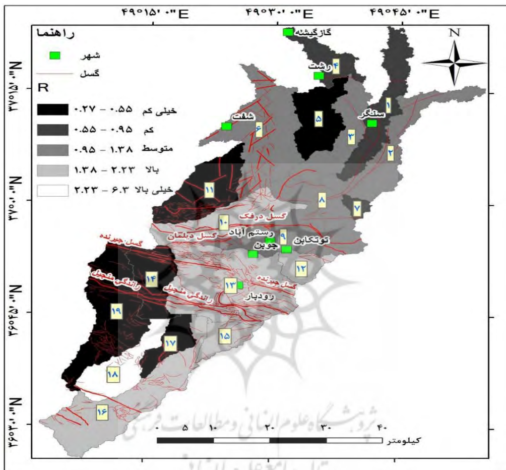
شکل ۶: نقشه‌ی پراکنده‌ی مقادیر شاخص انشعابات در منطقه‌ی مورد مطالعه.
