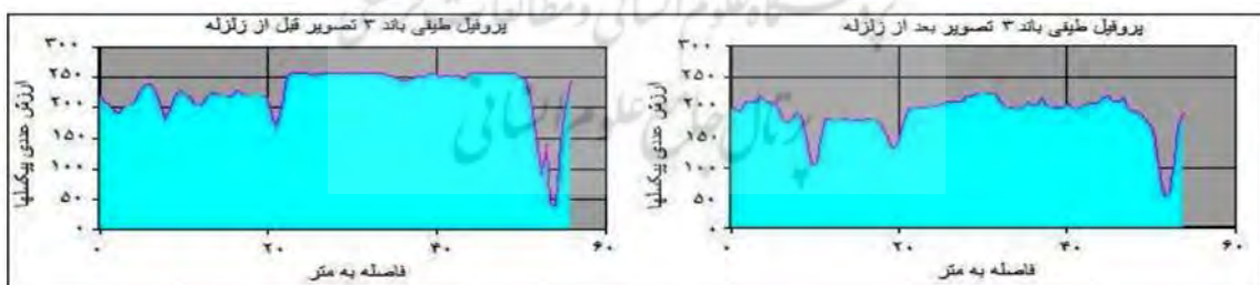
نگاره ۲۳: پروفیل بازتاب طیفی باند ۳
