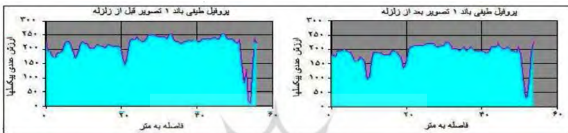
نگاره ۲۱: پروفیل بازتاب طیفی باند ۱
