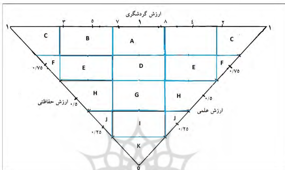
نمودار ۱. نمودار تعیین شرایط پایداری ژئومورفوسایت‌ها (منبع: اروجی، ۱۳۹۱)
