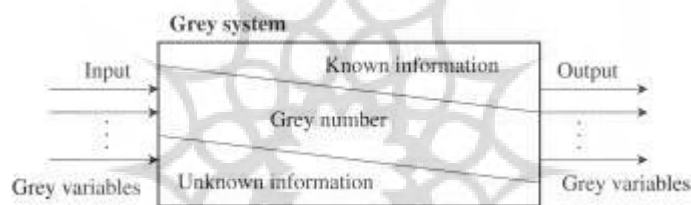
شکل ۱- مفهوم سیستم خاکستری (لی و همکاران، ۲۰۰۷، ۵۷۴)
