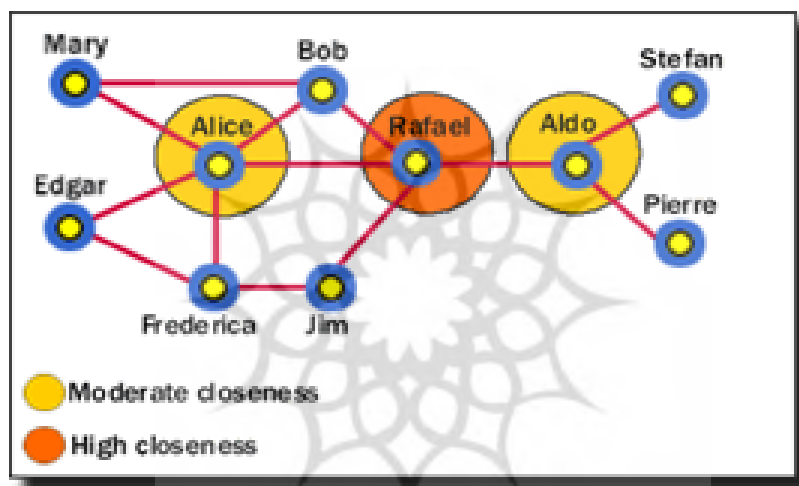
شکل ۴: شبکه‌ی نزدیکی مرکزیت عامل‌ها در یک شبکه (همان)
