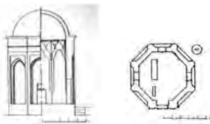
تصویر ۲. پلان، برش و نمای مقبره امامزاده جعفر اصفهان. مأخذ: www.Arthut.com
