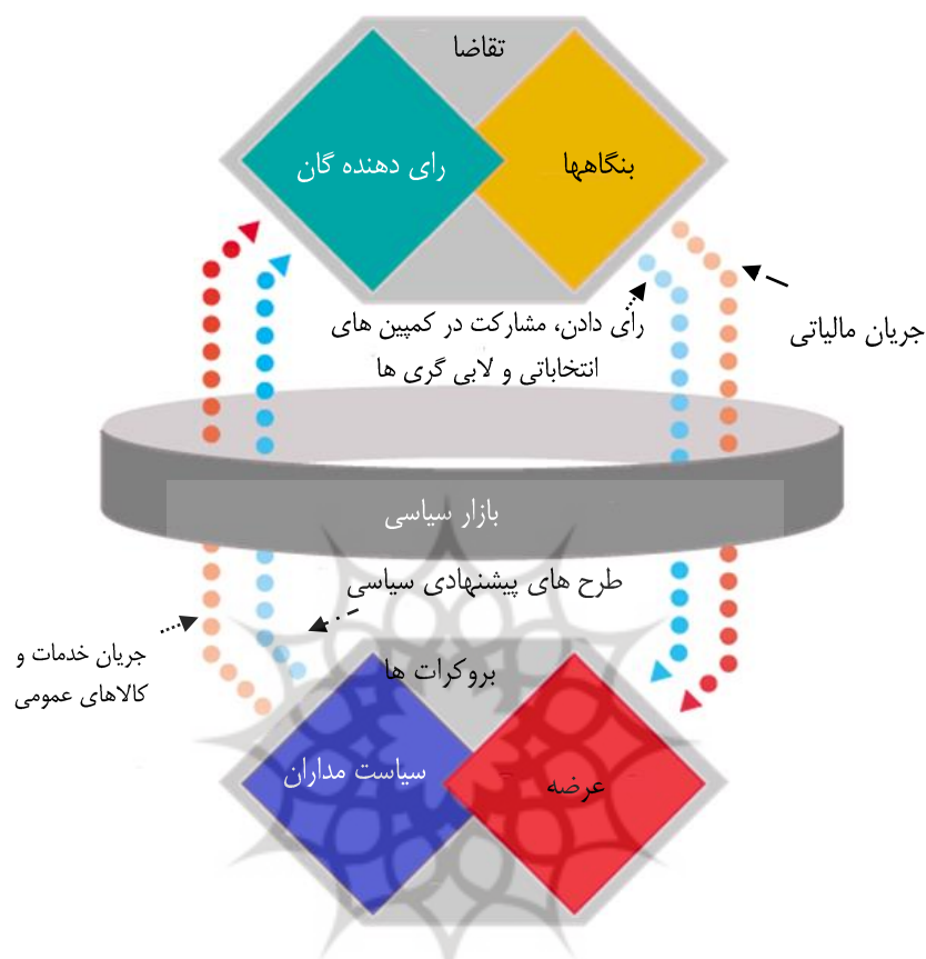
شکل ۱. بازار سیاسی و بازیگران آن
