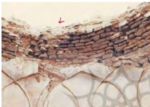
تصویر ۲۳. بقایای کاربردی گچی درون برج پاکار گنبد تخریب‌شده برج ینگگی ارخ (آ.م.ف. کردستان، ۱۳۶۲).
