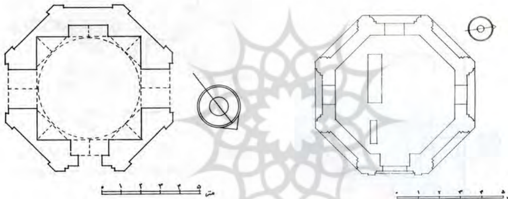
تصویر ۱۰. نقشه امامزاده جعفر قم در دوره ایلخانی (ویلیبر، ۱۳۶۵: ش ۱۰).
