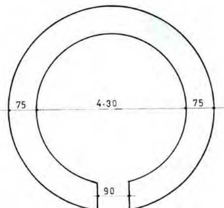
تصویر ۱۳. نقشه برج اوچ‌گنبدخان واقع در شهرستان بیجار (آ. م. ف. کردستان، ۱۳۶۳).
