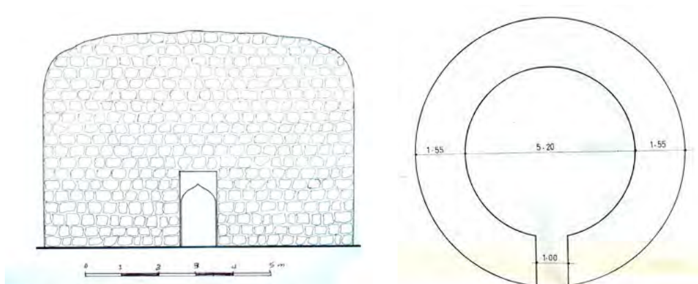
تصاویر ۱۹ و ۲۰. نقشه و نمای برج ینگه ارخ (آ.م. ف. کردستان، ۱۳۶۳).
