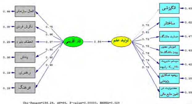
نمودار ۳. تحلیل مسیر دانشگاه کارآفرین باتولید علم در نظام آموزشی در حالت استاندارد
