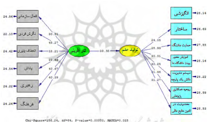
نمودار ۴. تحلیل مسیر دانشگاه کارآفرین باتولید علم در نظام آموزشی در حالت معنی دار
