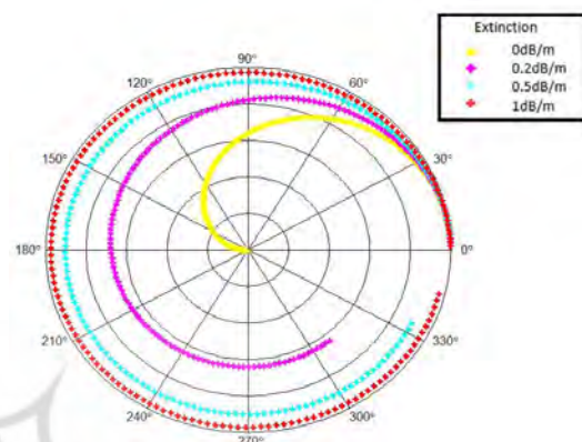
شکل ۹. نمایش مکان هندسی کوه‌رنسی حجمی در دایره مختلط واحد به‌ازای مقادیر متفاوت میرایی و ارتفاع لایه حجمی
