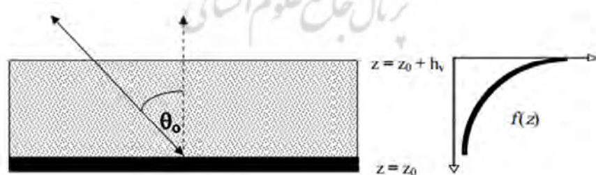
شکل ۵. تابع ساختار نمایی در مدل RVoG منبع: Cloude, 2005
