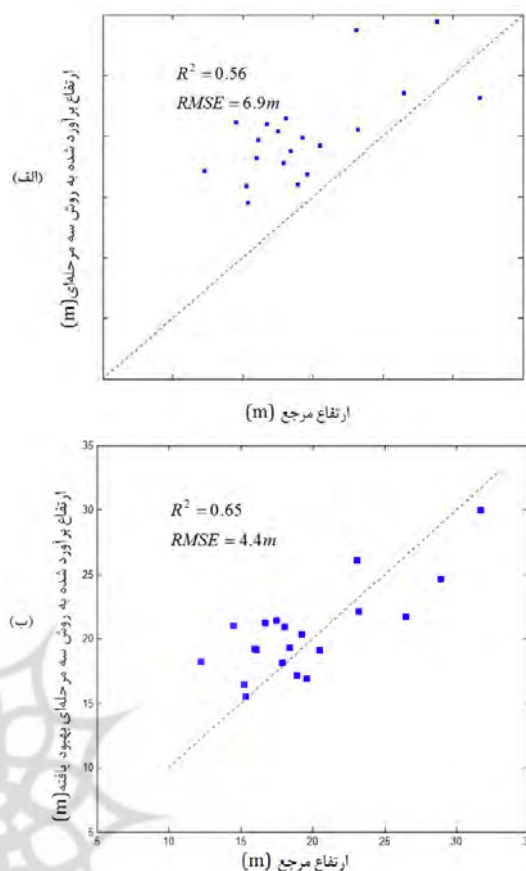
شکل ۱۲. مقایسه ارتفاع مرجع و ارتفاع برآورد شده با استفاده از تکنیک PolInSAR به روش: (الف) سه مرحله‌ای و (ب) سه مرحله‌ای بهبود یافته
