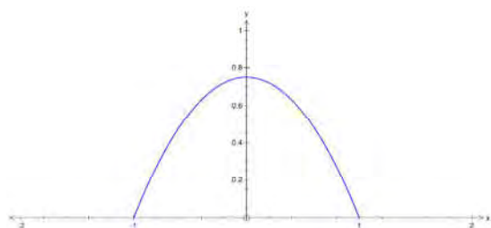
شکل ۱۲. تابع Epanechnikov
