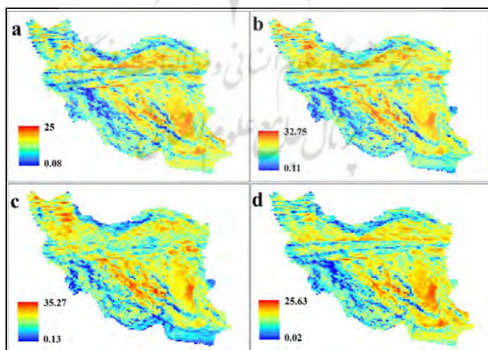
شکل (۳). قدر مطلق اختلافات بین دمای هوا و دمای سطحی در زمستان (a)، بهار (b)، تابستان (c) و پاییز (d) در دوره مطالعه.
