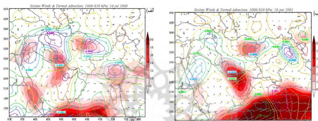
شکل ۲. بردارهای سرعت و جهت باد (m/s) و هسته‌های بیشینه سرعت باد (هاشورهای رنگی) تراز ۵۸۵۰ ه.پ؛ مجموع وزش دمایی (10^{-5} \text{s}^{-1}) \cdot \text{C}^{\circ} ترازهای ۹۲۵-۱۰۰۰ و ۸۵۰-۹۲۵ ه.پ؛ الف) الگوی همدید ۳، ۱۶ ژوئای ۲۰۰۸؛ ب) الگوی همدید ۴، ۲۸ ژوئن ۲۰۰۵
