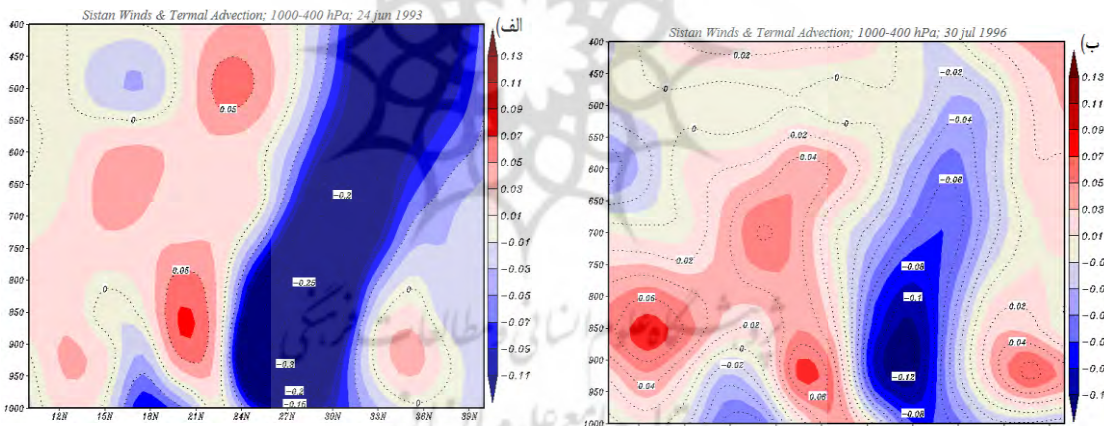
شکل ۷. نیمرخ ارتفاعی وزش دمایی جو ( 10^{-5} \text{K/s} ) از مدار 10^{\circ}N تا 40^{\circ}N در امتداد نصف‌النهار 60^{\circ}E ، از تراز ۴۰۰-۱۰۰۰ ه.پ؛ الف) الگوی همدید ۱، ۲۴ ژوئن ۱۹۹۳؛ ب) الگوی همدید ۲، ۳۰ ژوئیه ۱۹۹۶
