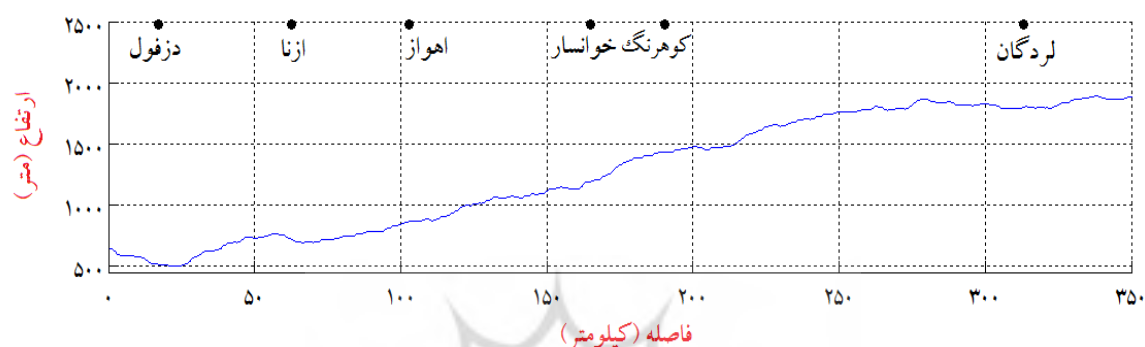
شکل ۱۳. آهنگ تغییرات شمار روزهای برف‌پوشان و ارتفاع در راستای غرب به شرق (برف‌خوآن زاگرس)
