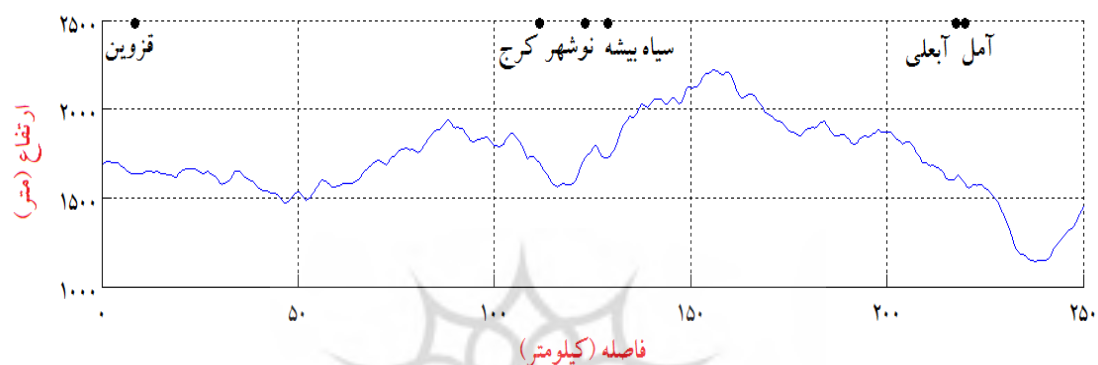
شکل ۳. آهنگ تغییرات شمار روزهای برف‌پوشان و ارتفاع در راستای غرب به شرق (برف‌خوان البرز)
