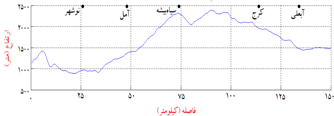
شکل ۴. آهنگ تغییرات شمار روزهای برف‌پوشان و ارتفاع در راستای شمال به جنوب (برف‌خوان البرز)
