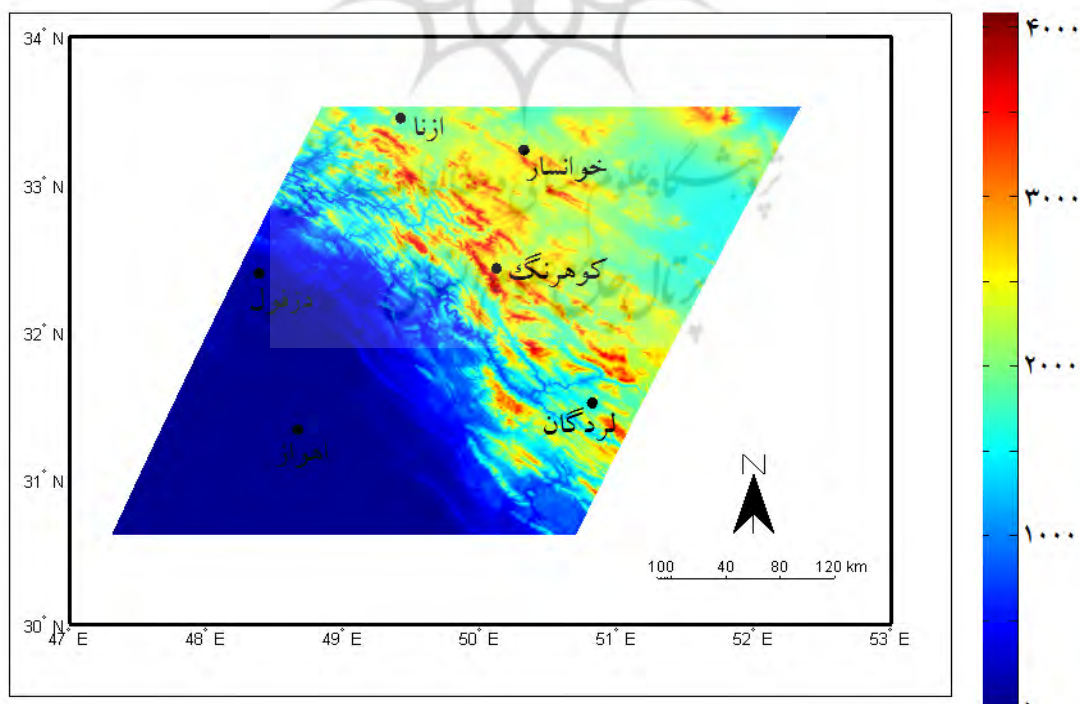
شکل ۱۲. نقشه مدل رقمی ارتفاع برف‌خون زاگرس (ارتفاع - متر)
