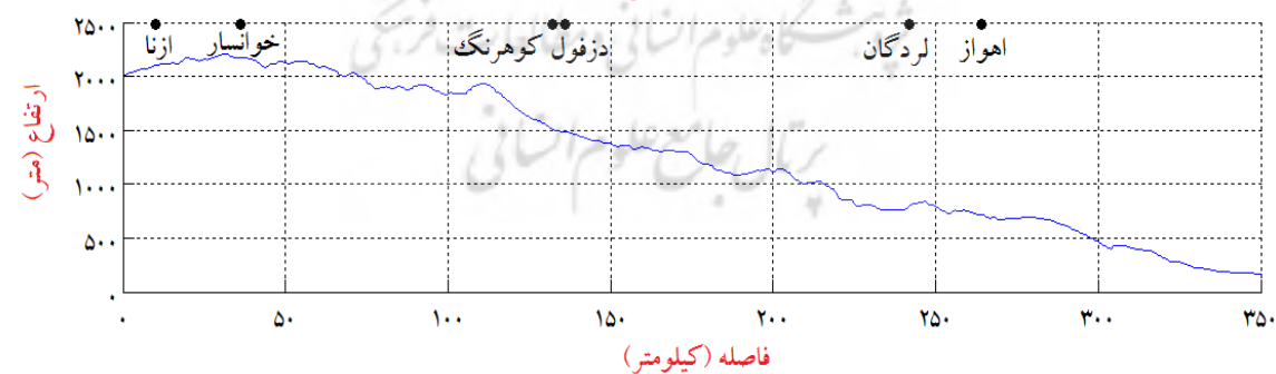
شکل ۱۴. آهنگ تغییرات شمار روزهای برف‌پوشان و ارتفاع در راستای شمال به جنوب (برف‌خوآن زاگرس)
