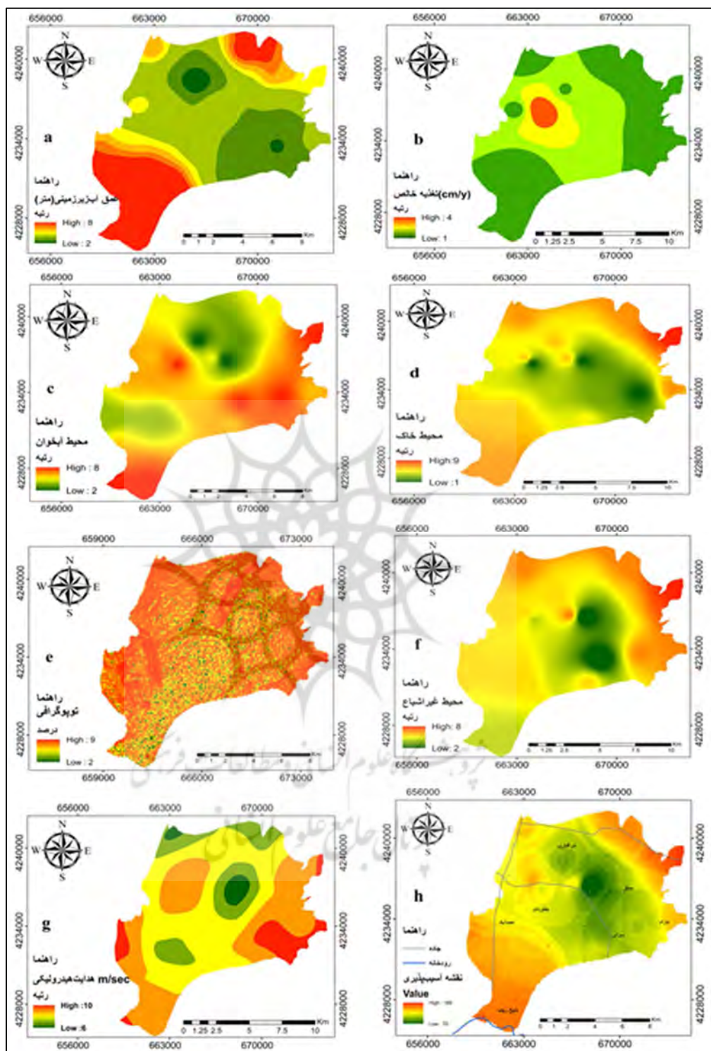
شکل ۵: نقشه پهنه‌بندی پارامترهای SINTACS (a؛ عمق آب زیرزمینی؛ b تغذیه؛ c محیط آبخوان؛ d محیط خاک؛ e توپوگرافی؛ f محیط غیرانواع؛ g هدایت هیدرولیکی؛ h نقشه آسیب‌پذیری
