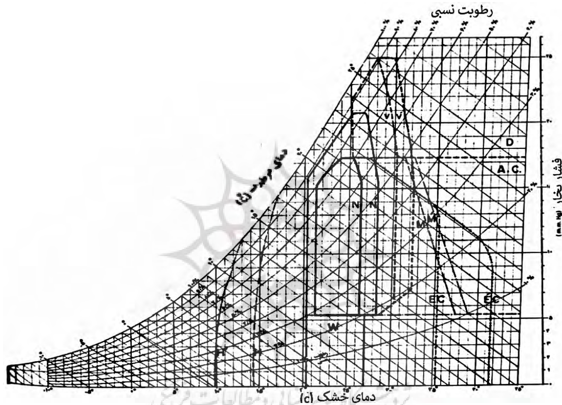
شکل شماره ۲: نمودار بیوکلیماتیک ساختمانی گیونی (Givoni, 1989)
