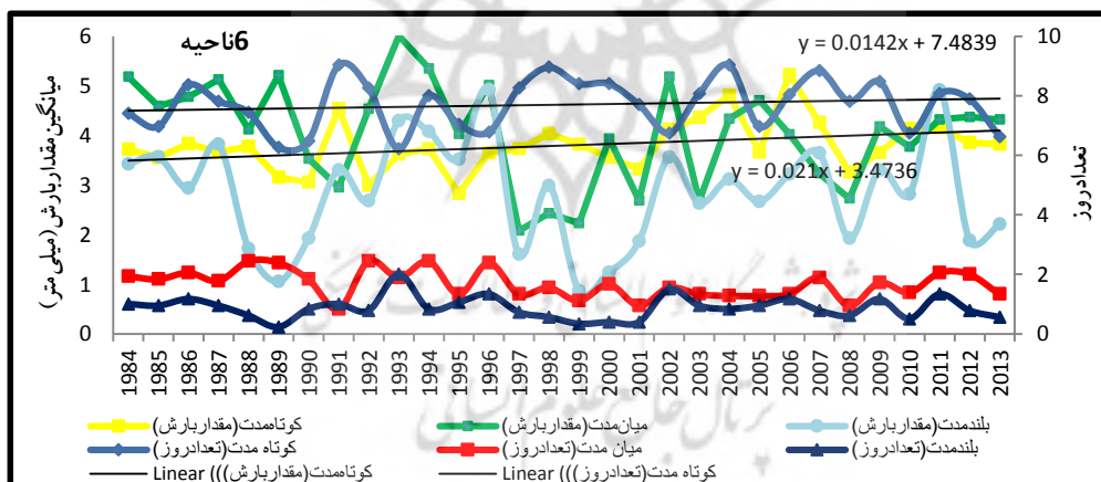
شکل ۸. نمودار تعداد روز بارشی و میانگین بارش روزانه ناحیه ۶
