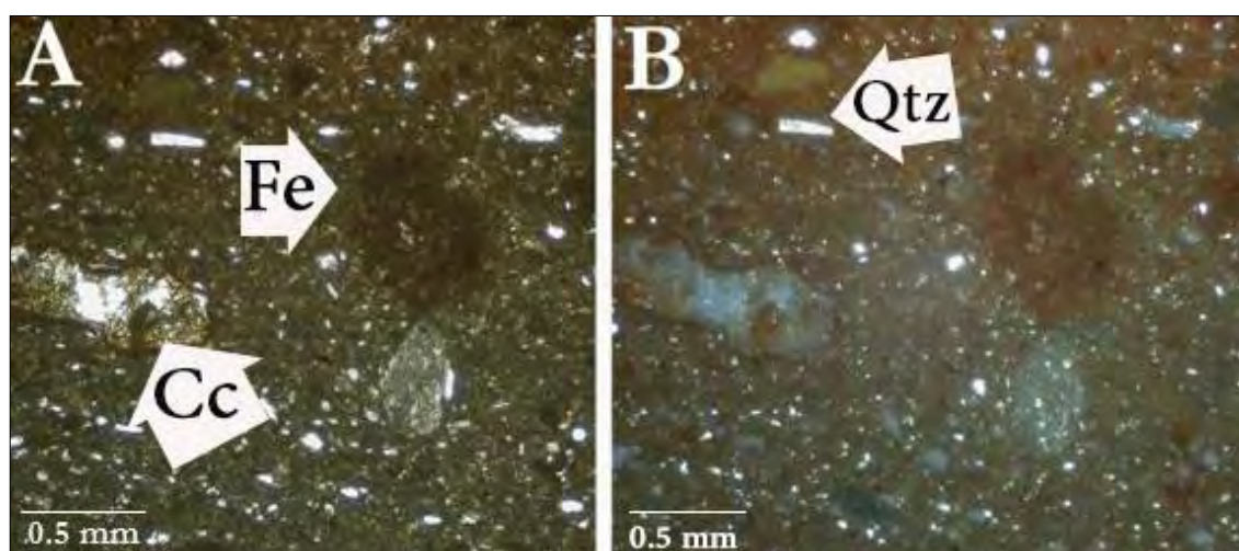
شکل ۸: تصاویر میکروسکوپی خمره زیستی، طول میدان دید 2.7 mm، بزرگنمایی ۴۰۰ برابر، تصویر سمت راست B نور XPL و تصویر سمت چپ A نور PPL، بافت سیلتی، آهن کلئیدی با رنگ قرمز-قهوه‌ای، Qtz: کانی کوارتز با رنگ روشن، ریزبلور و فراوان به صورت شناور در زمینه رسی دیده می‌شود، Cc: کلسیت ثانویه.
