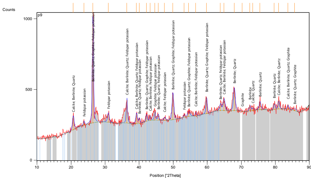
شکل ۹: دیاگرام XRPD نمونه مورد نظر، نشان‌دهنده‌ی فازهای کوارتز، گرافیت، برلینیت، کلسیت و فلدسپار پتاسیم است.
