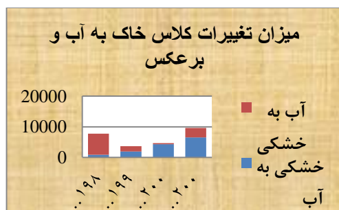
شکل ۱۰. نمودار میزان تبدیلات کلاس ها در هر چهار دوره
