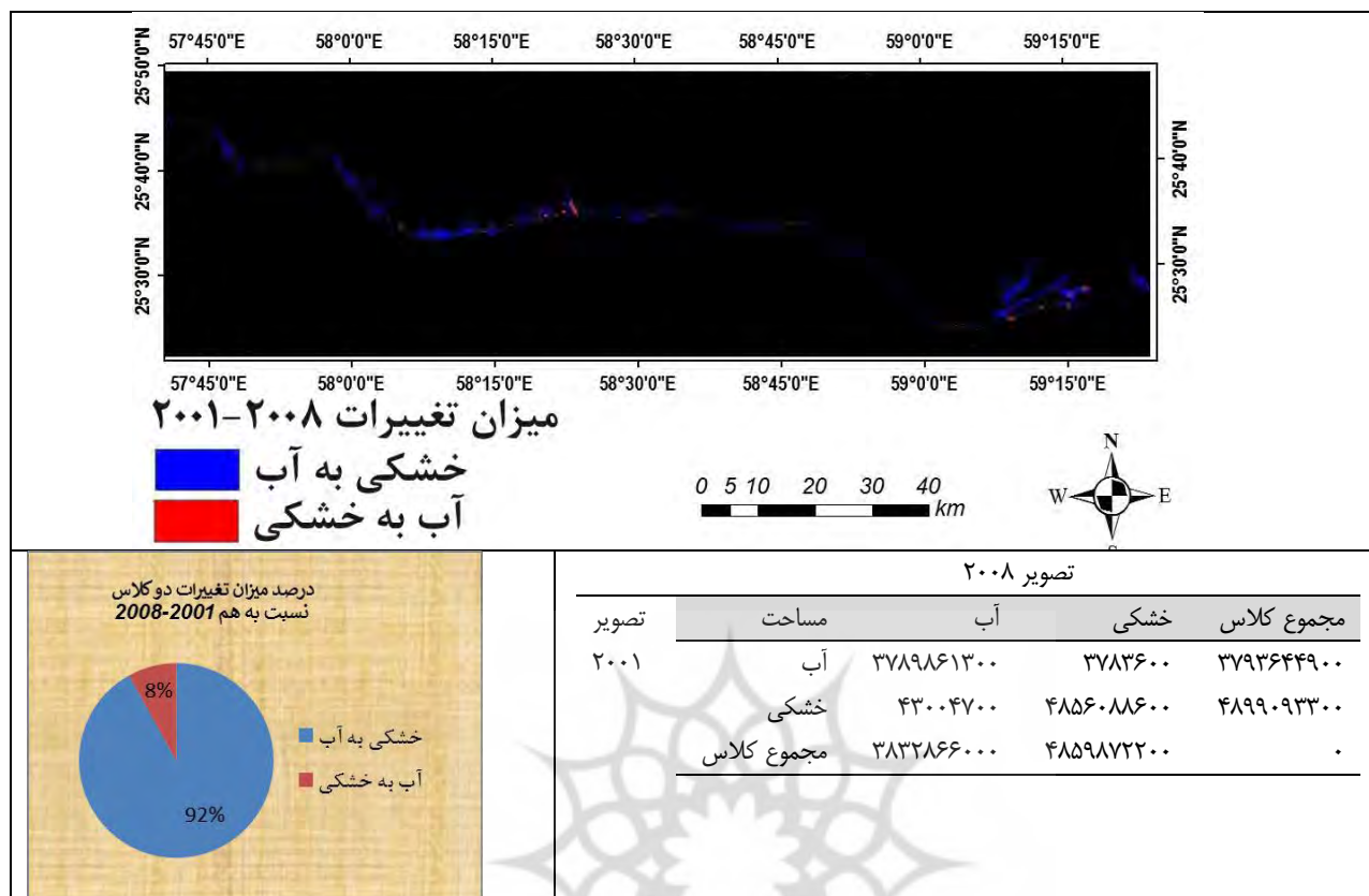
شکل ۸. الف) تصویر، ب) اطلاعات from-to، و ج) نمودار مساحت (درصد) میزان تبدیلات دو کلاس آب و خشکی حاصل از detection change منطقه مورد مطالعه از ۲۰۰۸-۲۰۰۱
