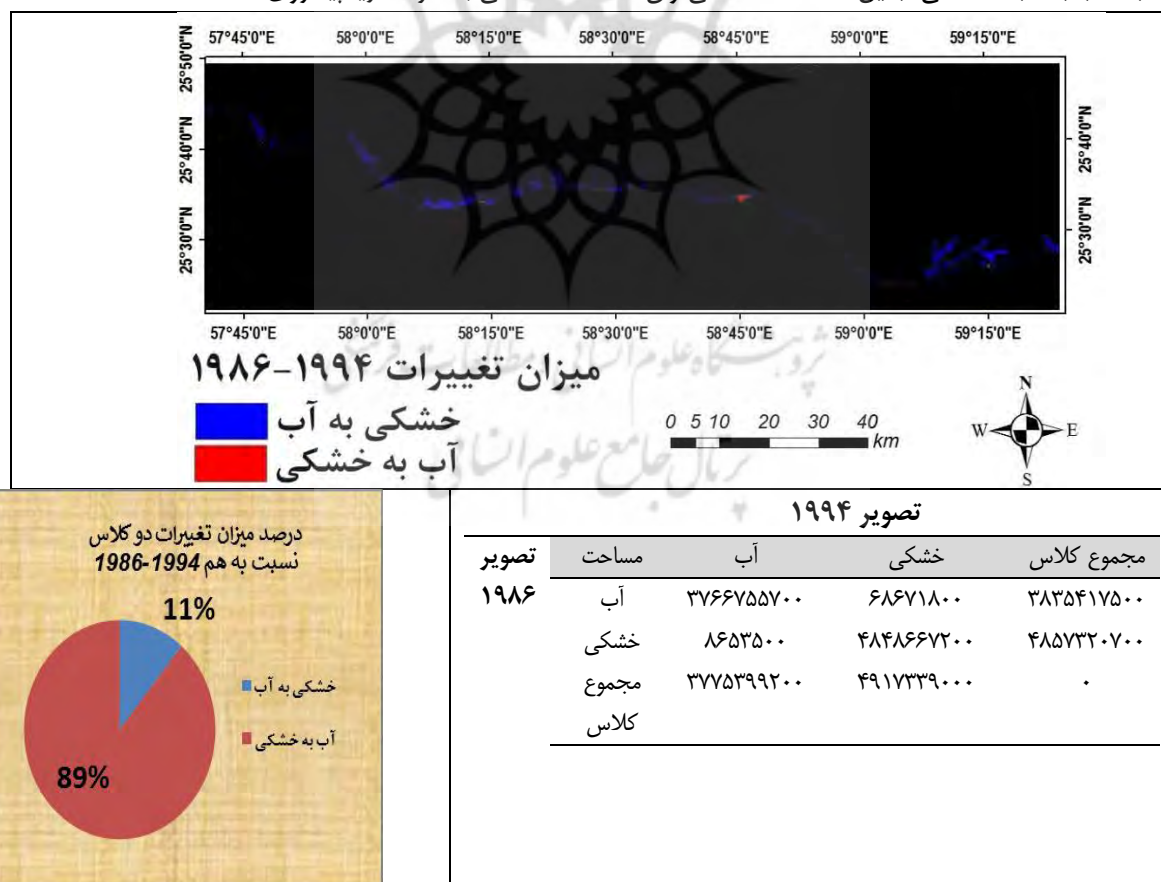
شکل ۶. الف) (تصویر، ب) اطلاعات from-to، و ج) نمودار مساحت (درصد) میزان تبدیلات دو کلاس آب و خشکی حاصل از change detection منطقه مورد مطالعه از دوره ۱۹۸۶-۱۹۹۴
