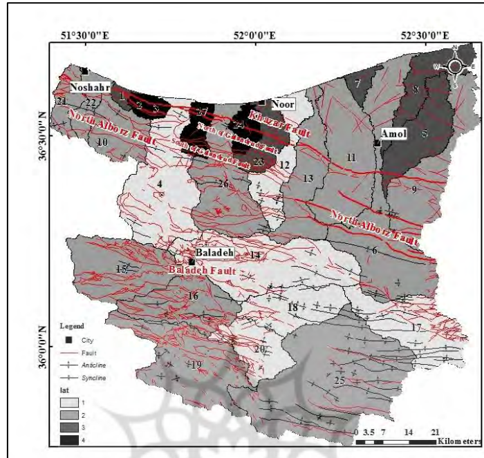
شکل ۱۳: نقشه ی توزیع سطح فعالیت زمین ساخت نسبی (lat) در منطقه ی مورد مطالعه
