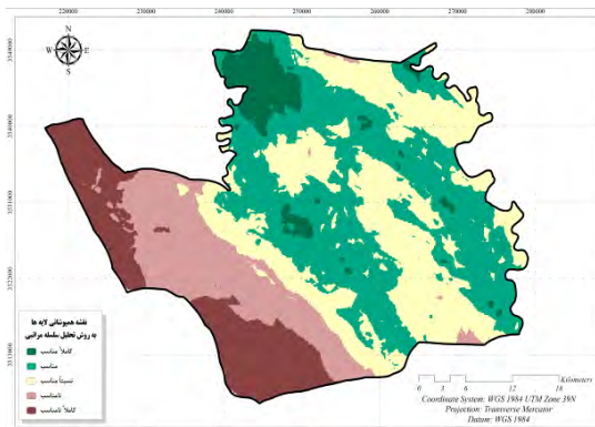
شکل ۲۳- نقشه تعیین اولویت نهایی براساس مدل AHP
