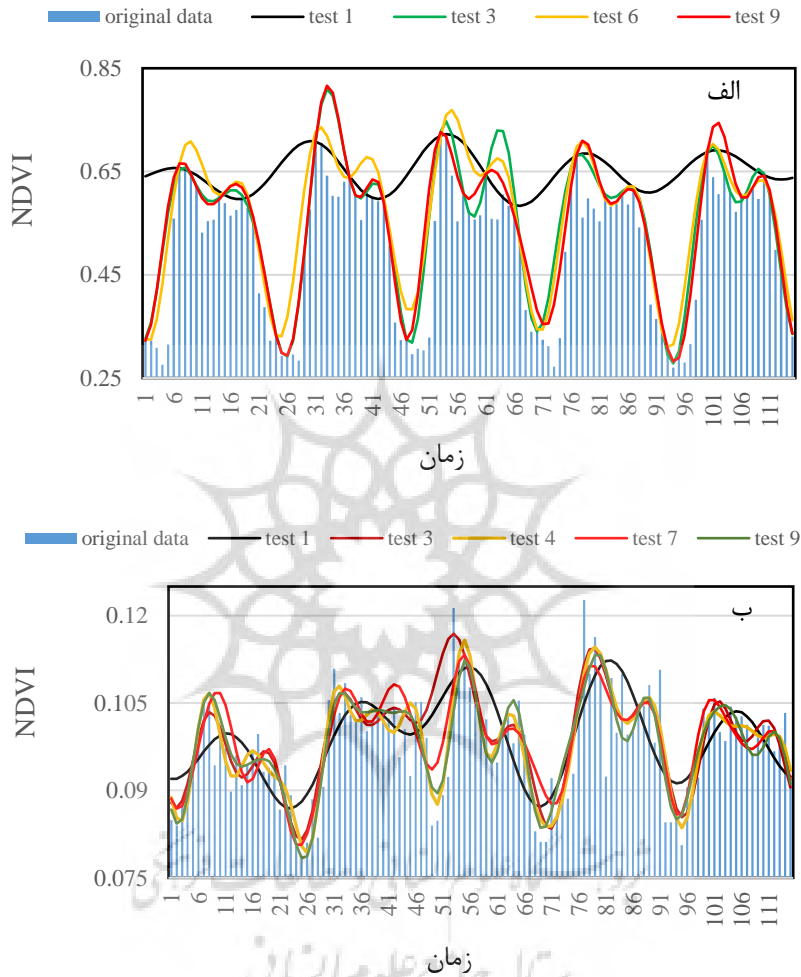
شکل ۵ نتایج حاصل از الگوریتم HANTS بر روی باغات (الف)، تیپ مرتعی Ar. sieberi (ب)
