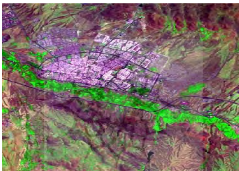
شکل ۱. تصویر ماهواره‌ای لندست ۵ (۱۳۸۵)
