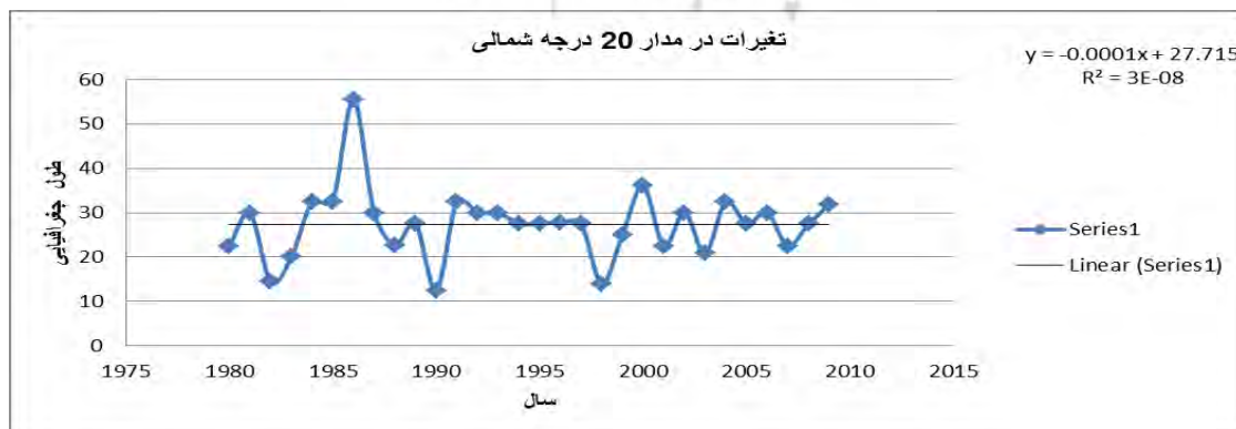
شکل ۳. تغییرات ناوه مدیترانه در مدار ۲۰ درجه شمالی
