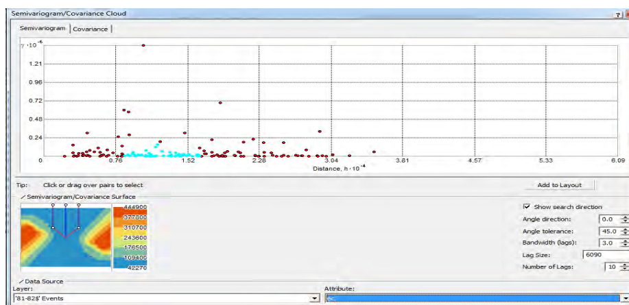
شکل ۶- مقادیر سمی واریوگرام پارامتر EC از مرکز به شمال دشت و توزیع نقاط زوج با فاصله کم و تغییرات بالا
