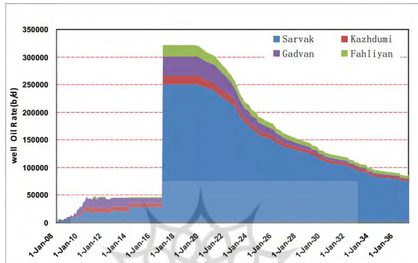
نمودار 1- پروفایل پیشنهادی تولید میدان آزادگان جنوبی
