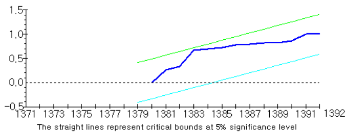
شکل (۲): آزمون ثبات ساختاری با روش پسماند تجمعی منبع: یافته‌های تحقیق
