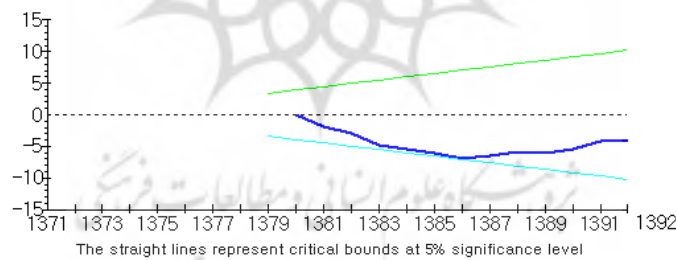
شکل (۱): نتایج آزمون ثبات ساختاری با روش محاسبه آماره پسماند تجمعی منبع: یافته‌های تحقیق
