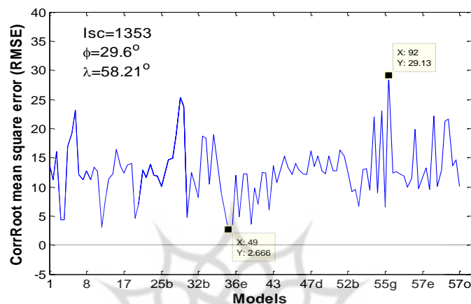
شکل ۴) مقادیر ریشه میانگین مربعات خطا محاسبه شده برای مدل‌ها (RMSE)
