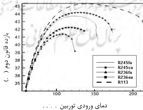
شکل ۵) بازده قانون دوم سیستم در مقابل دمای ورودی توربین برای سیالات کارکن در سه گروه A، B و C
