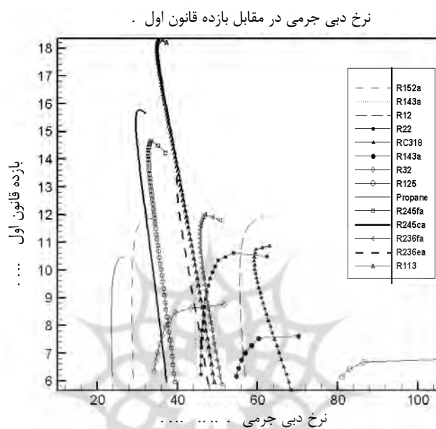
شکل ۸) بازدهی گرمایی سیستم در مقابل نرخ دبی جرمی برای سیالات کارکن
