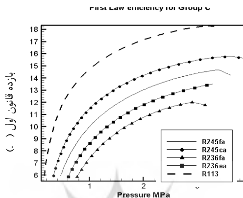
شکل ۶) راندمان حرارتی سیستم در مقابل فشار اواپراتور برای سیالات کارکن در سه گروه A، B و C نرخ دبی جرمی برای گروه .
