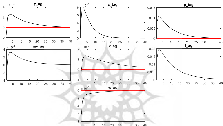
شکل (۳) تابع‌های واکنش آنی متغیرهای بخش کشاورزی در برابر تکانه عرضه نیروی کار
