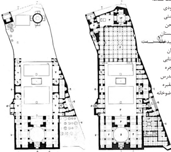
تصویر ۱. پلان‌های مسجد-مدرسه رحیم خان. مأخذ: حاجی قاسمی، ۱۳۷۵.
