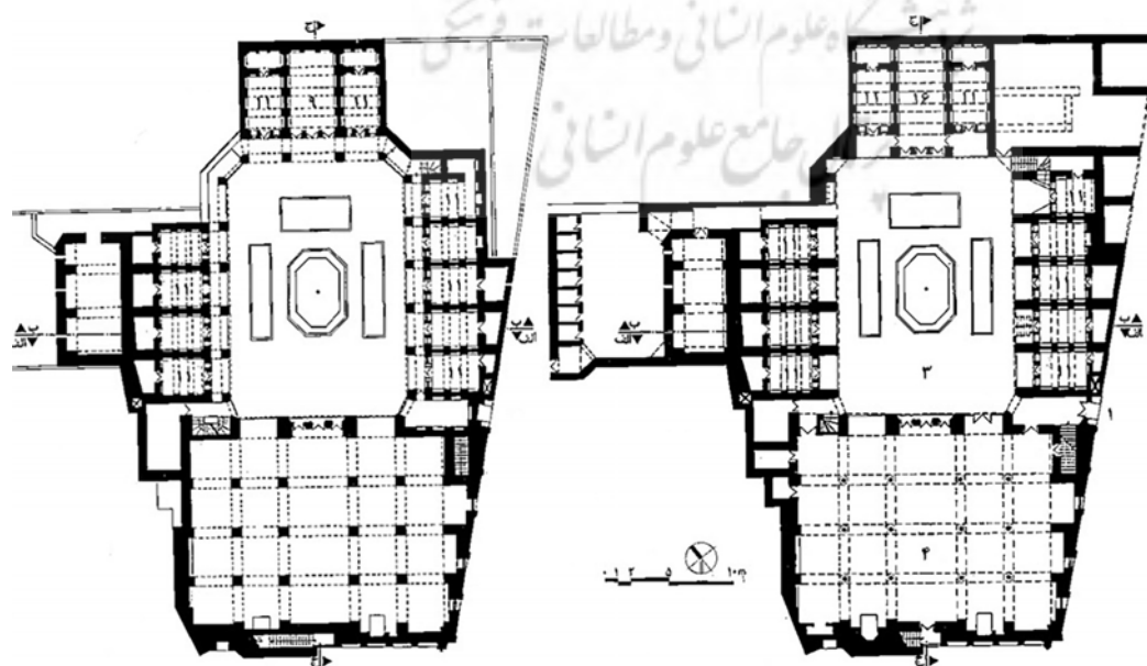
تصویر ۳. پلان‌های مسجد-مدرسه معمارباشی. مأخذ: حاجی قاسمی، ۱۳۷۵.
