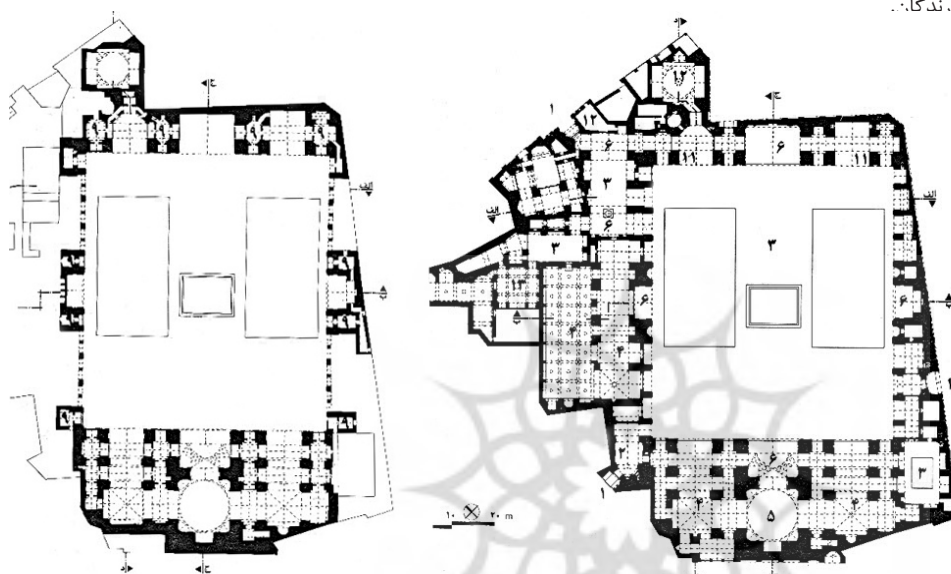
تصویر ۲. پلان‌های مسجد-مدرسه حکیم. مأخذ: حاجی قاسمی، ۱۳۷۵.
