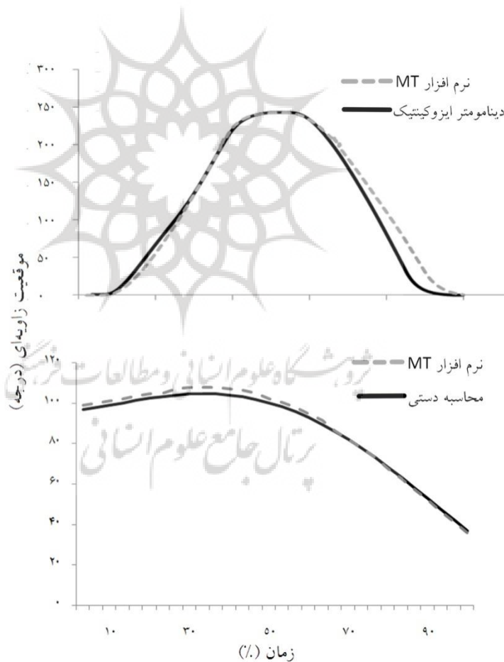
شکل ۷. نمودار موقعیت زاویه ای - زمان؛ مقایسه MT با دینامومتر ایزوکینتیک در تحلیل دوبعدی (بالا)، مقایسه MT با محاسبه دستی زاویه زانو در تحلیل سه بعدی (پایین)
