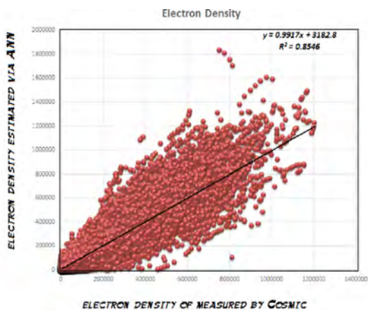
نگاره ۳: نمودار رگرسیون مدل‌سازی چگالی الکترون ماهواره‌ی COSMIC
